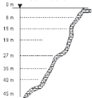
Schnitt a-a
